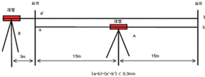
그림 1. 전자레벨 점검
